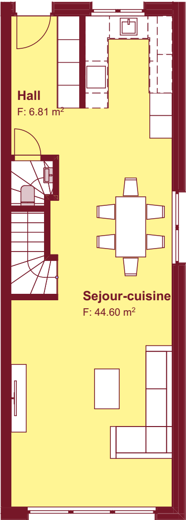
0. Erdgeschoss 1:100
